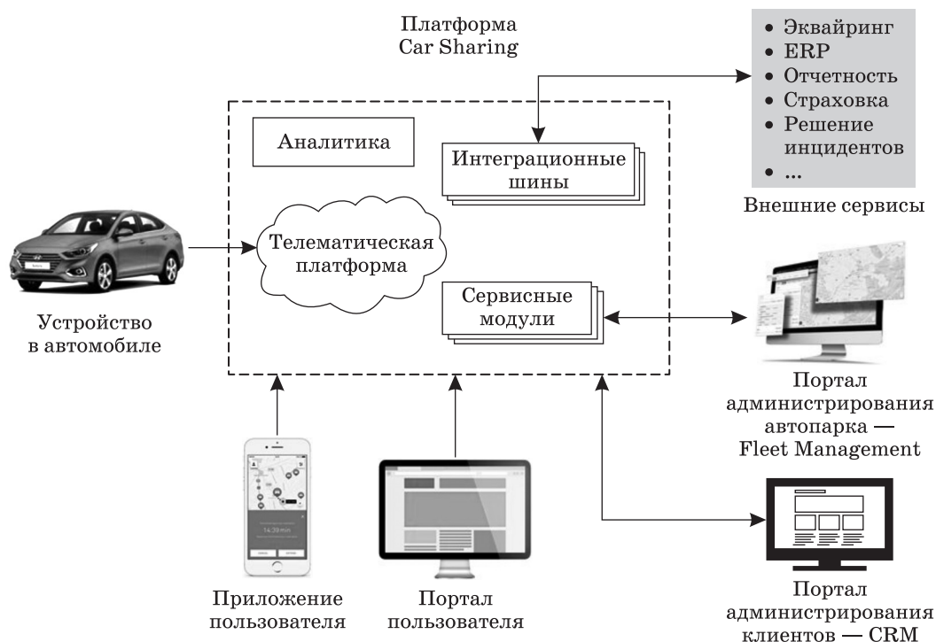
Рис. 1. Технологическая архитектура каршеринга
